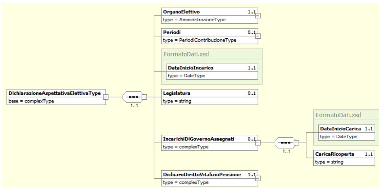
Figura 2: DichiarazioneAspettativaElettivaType
