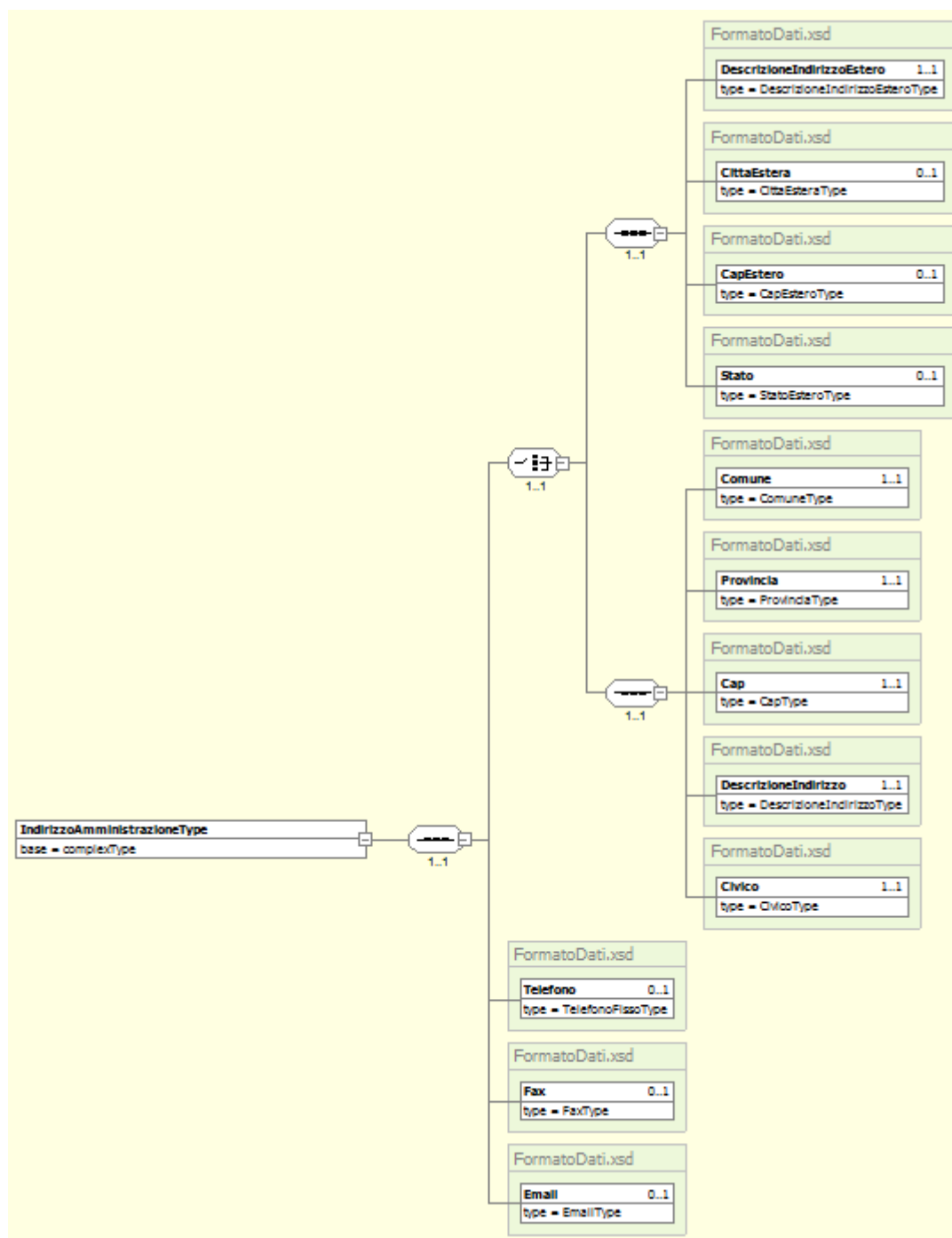
Figura 5 - IndirizzoAmministrazione Type
