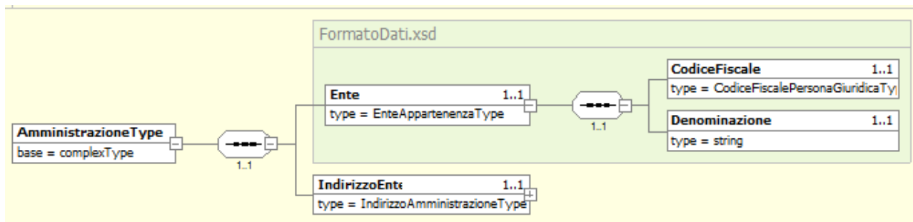
Figura 4: AmministrazioneType
