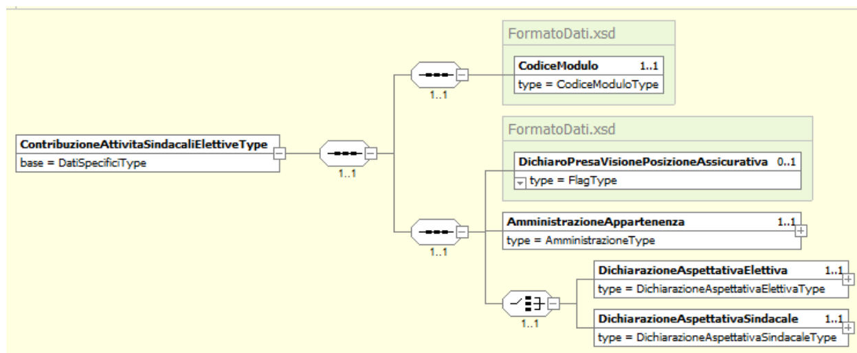
Figura 1 – ContribuzioneAttivitaSindacaliElettiveType
