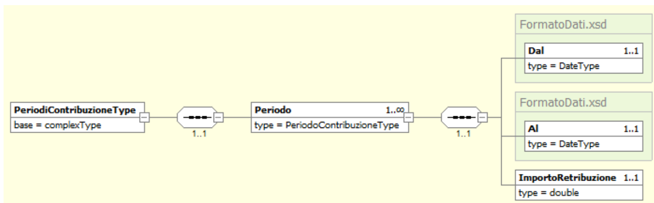
Figura 6: PeriodiContribuzioneType
