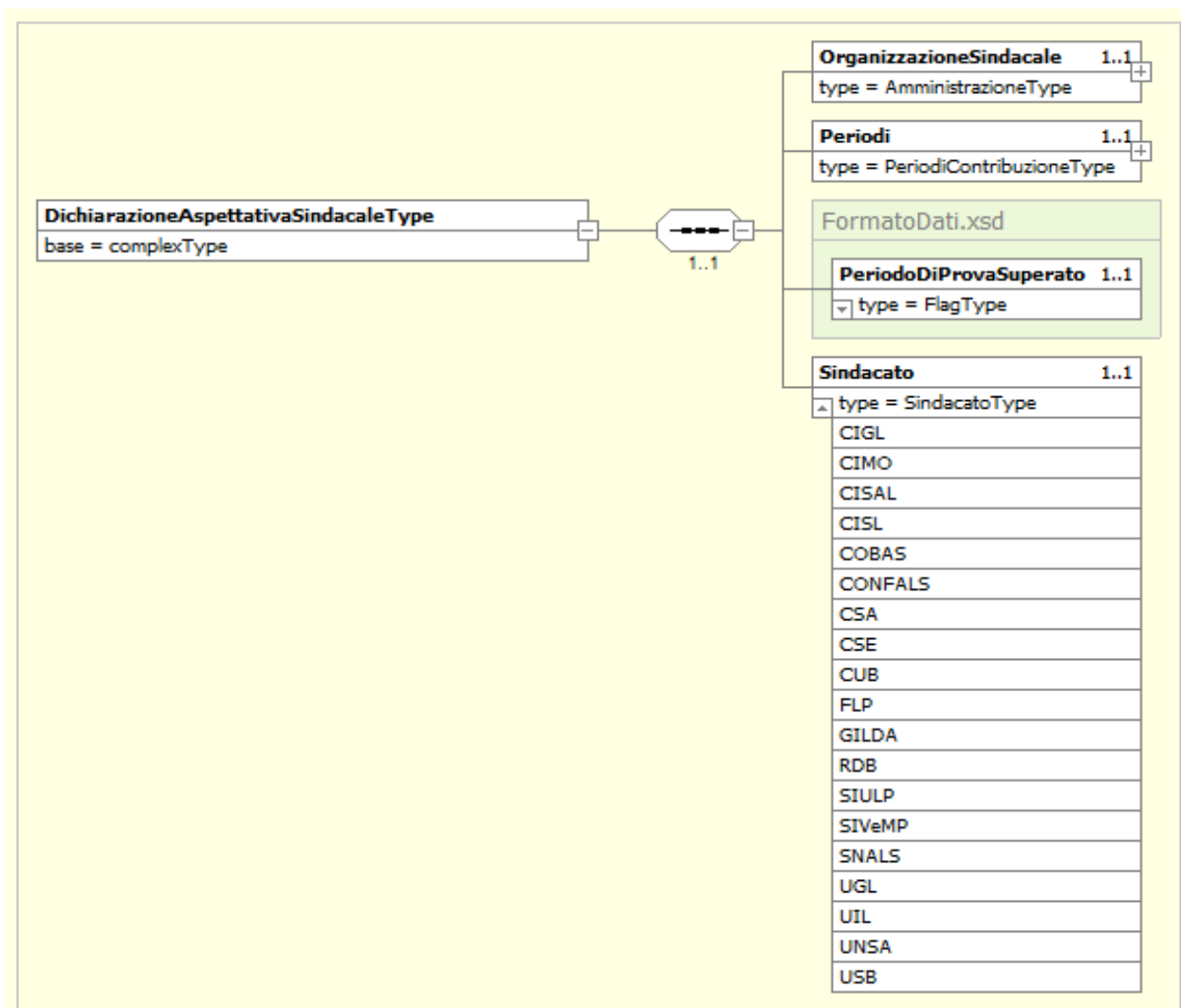
Figura 3: DichiarazioneAspettativaSindacaleType
