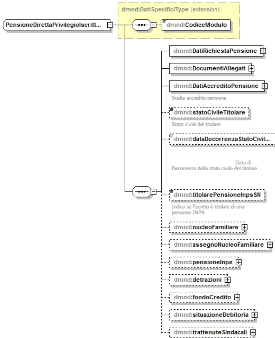
Figura 4 - PensioneDirettaPrivilegiolscritto.xsd
