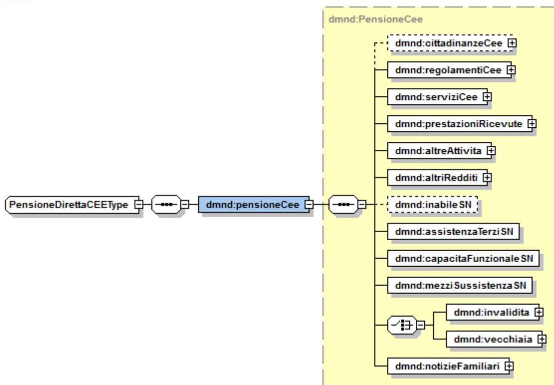
Figura 2 - PensioneDirettaCEE.xsd
