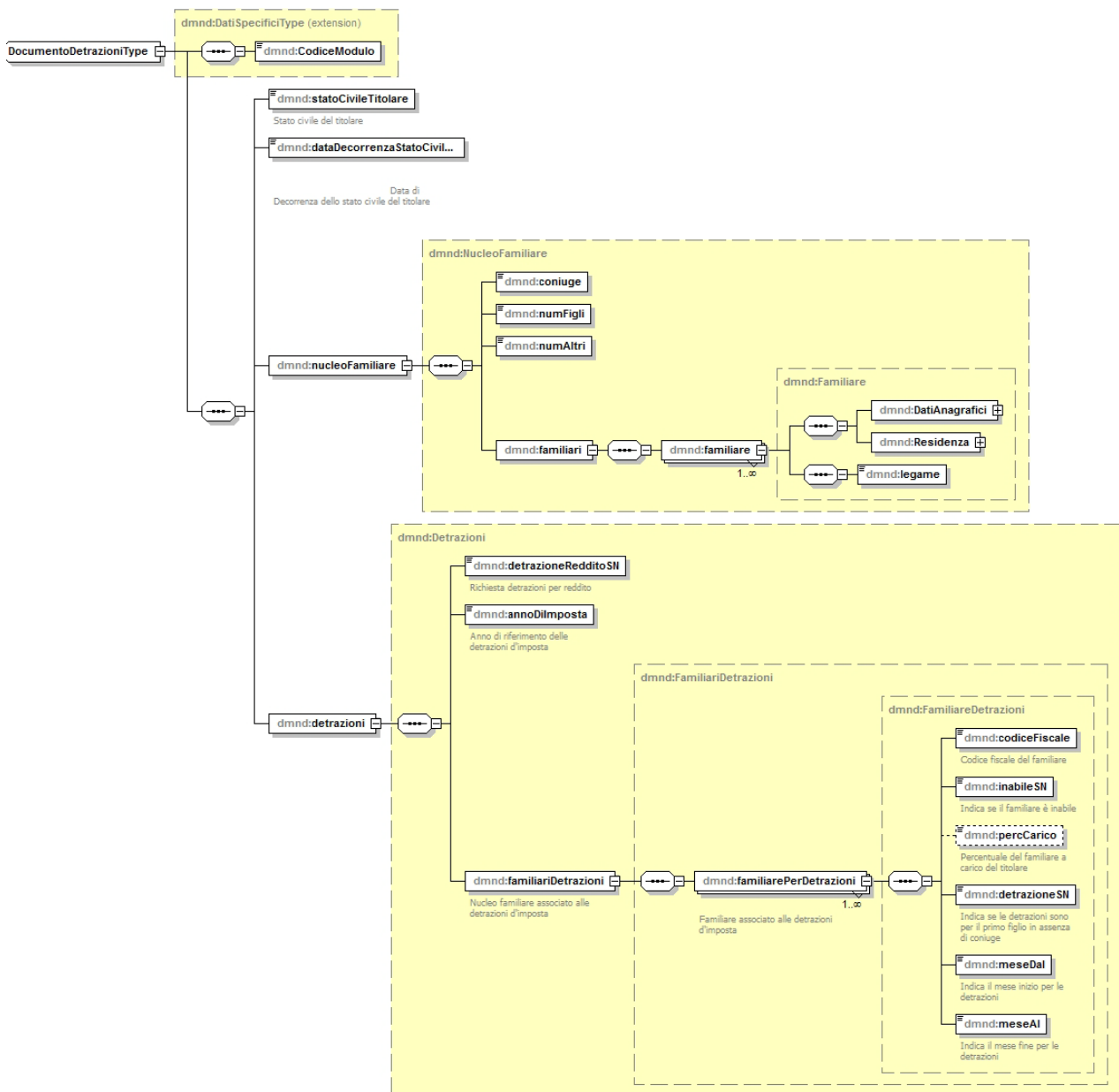
Figura 5 - VIN_DocumentoDetrazioni.xsd
