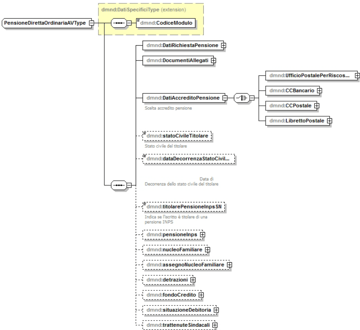
Figura 1 - PensioneDirettaOrdinariaAV.xsd
