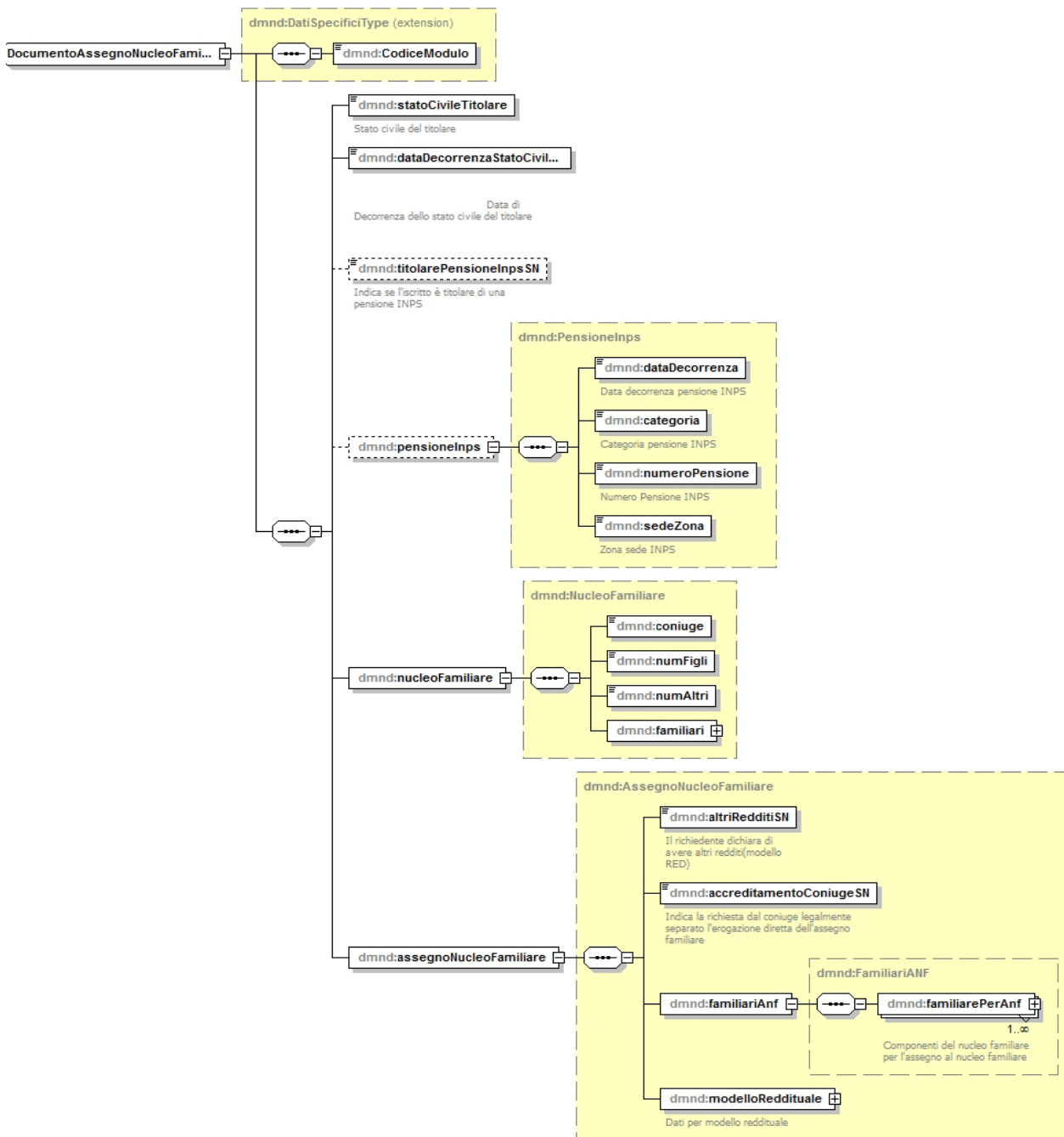
Figura 6 - VIN_DocumentoAssegnoNucleoFamiliare.xsd
