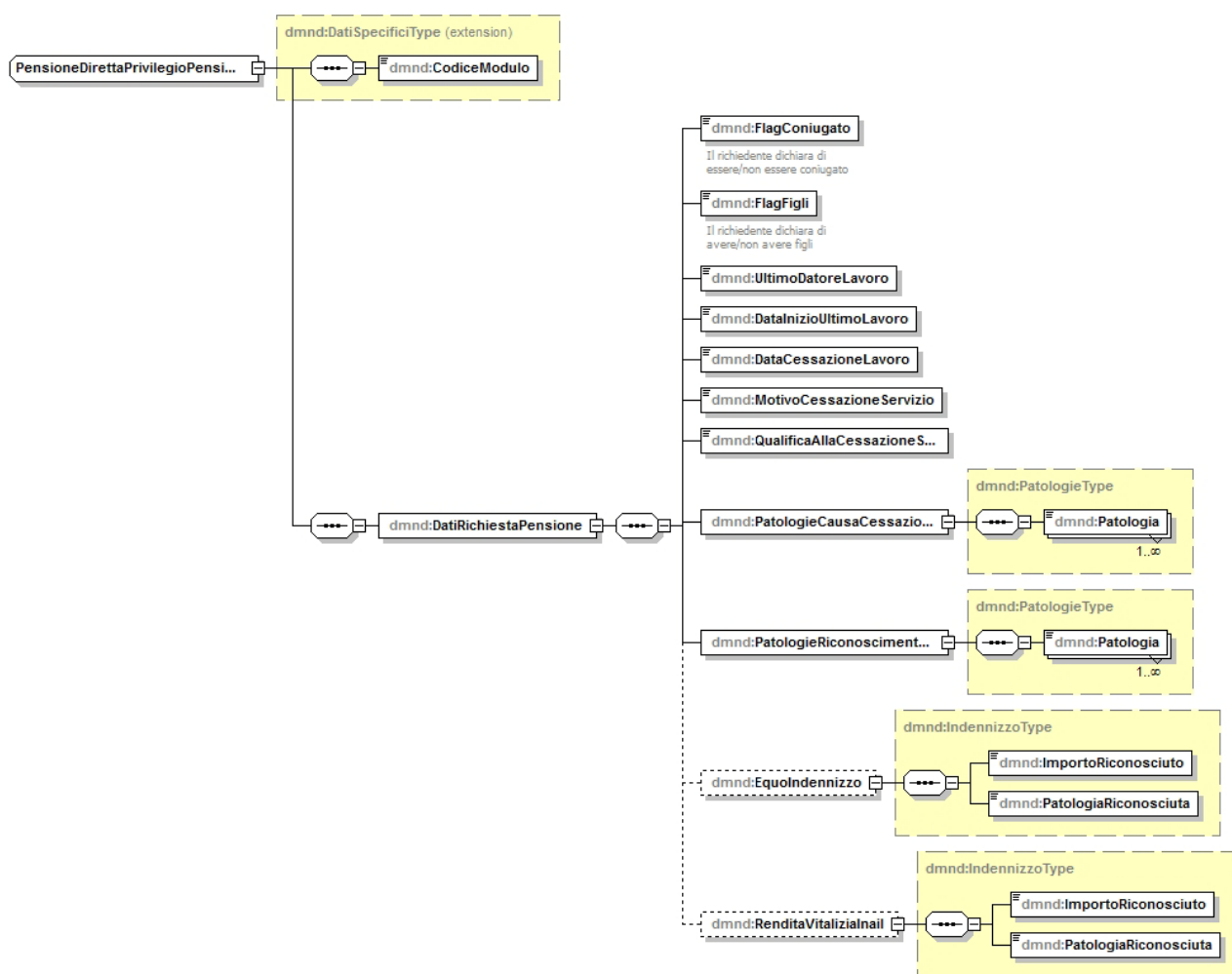
Figura 3 - PensioneDirettaPrivilegioPensionato.xsd
