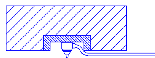
PARTICOLARE TESTINA NEL SOFFITTO scala 1:10
