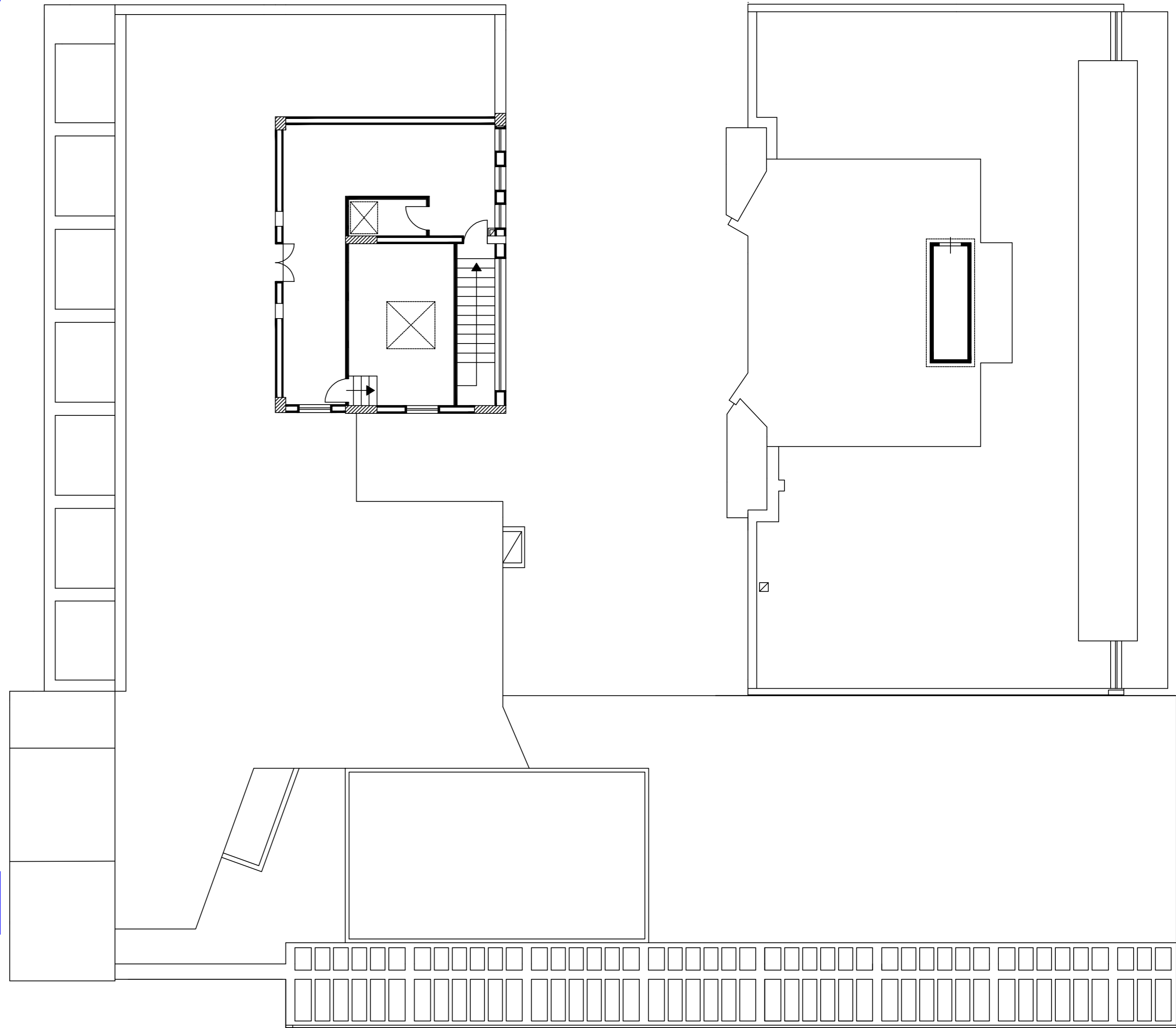
PIANO COPERTURA
