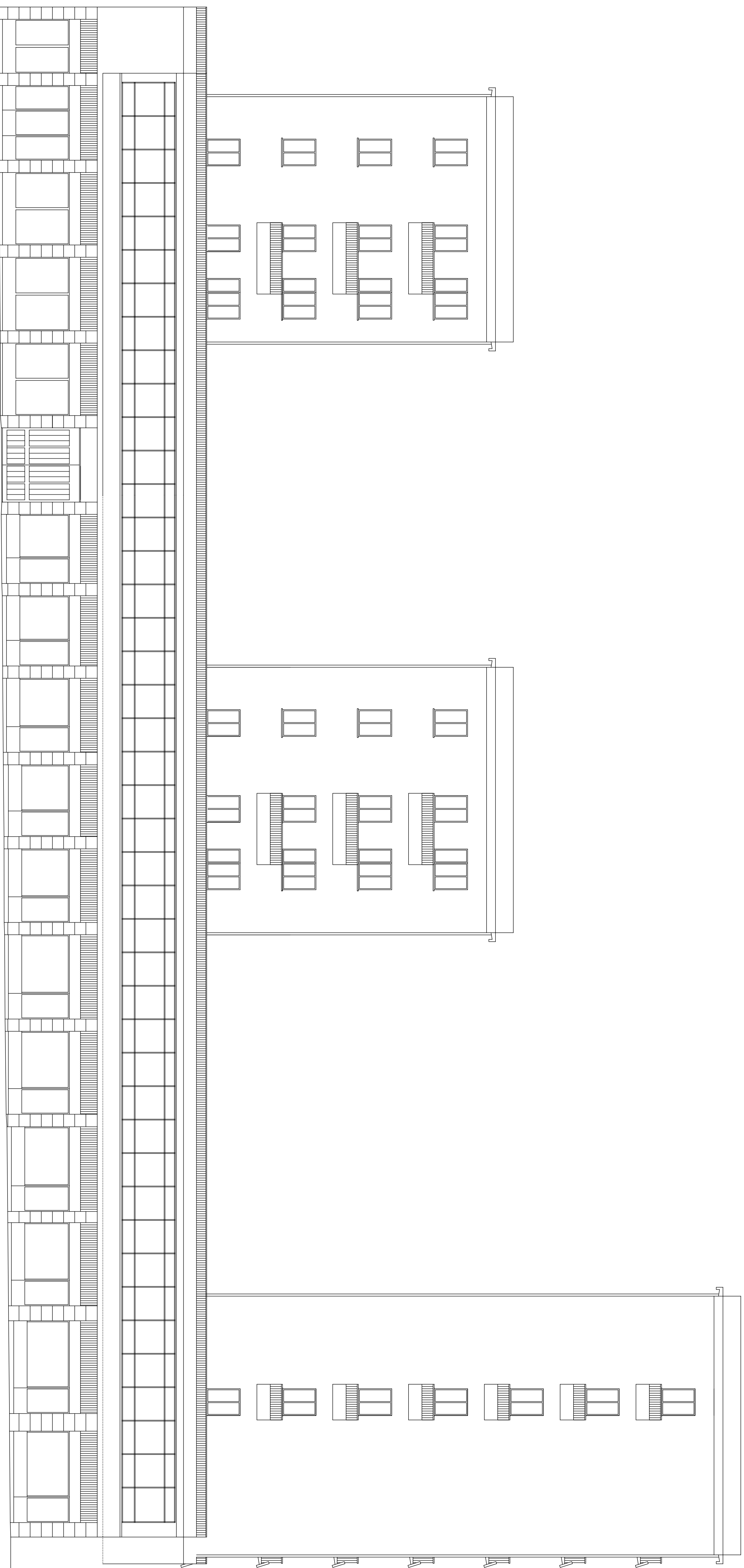
PROSPETTO NORD (VIA G.B. VICO)
