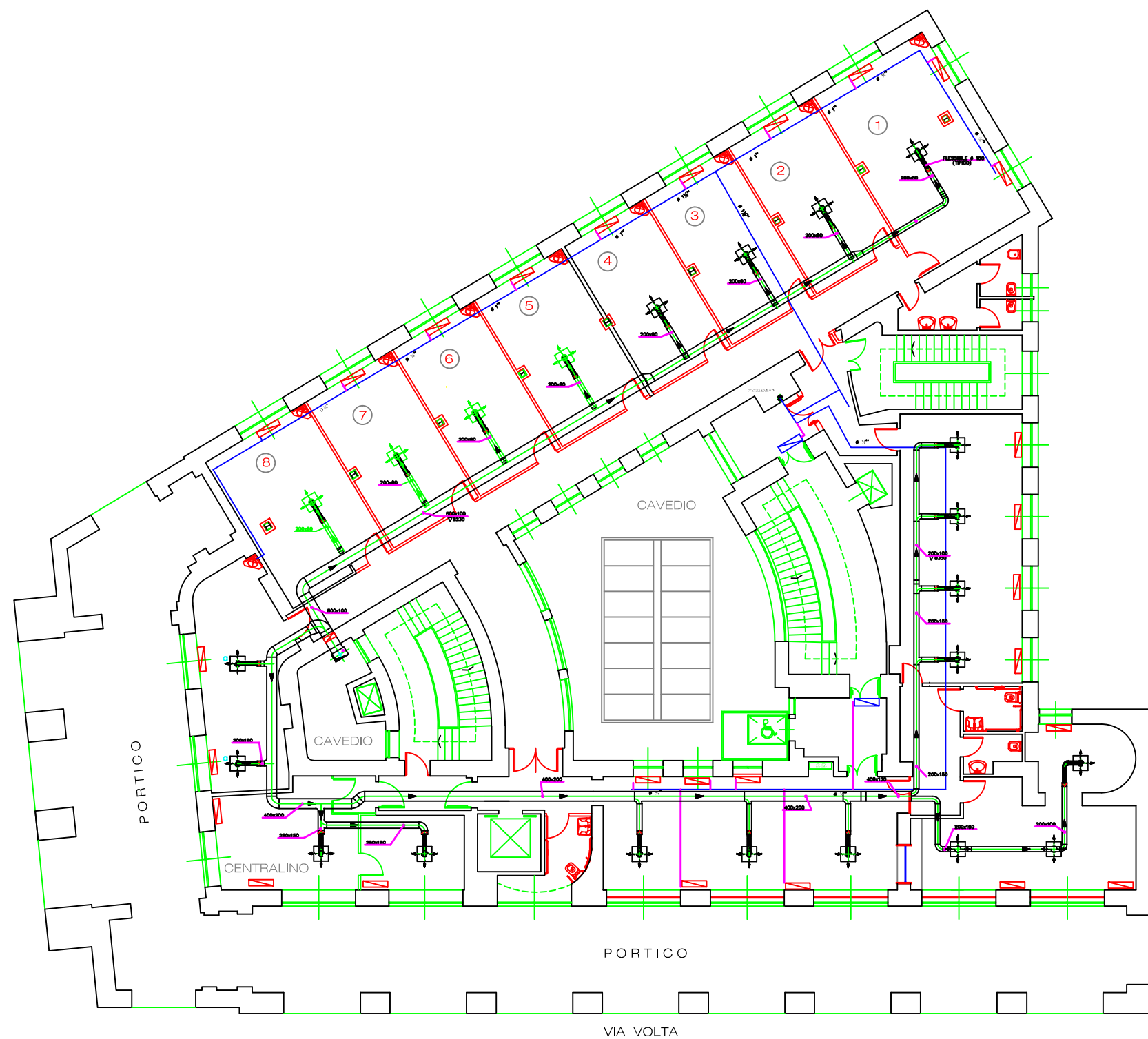
PIANTA PIANO AMMEZZATO
