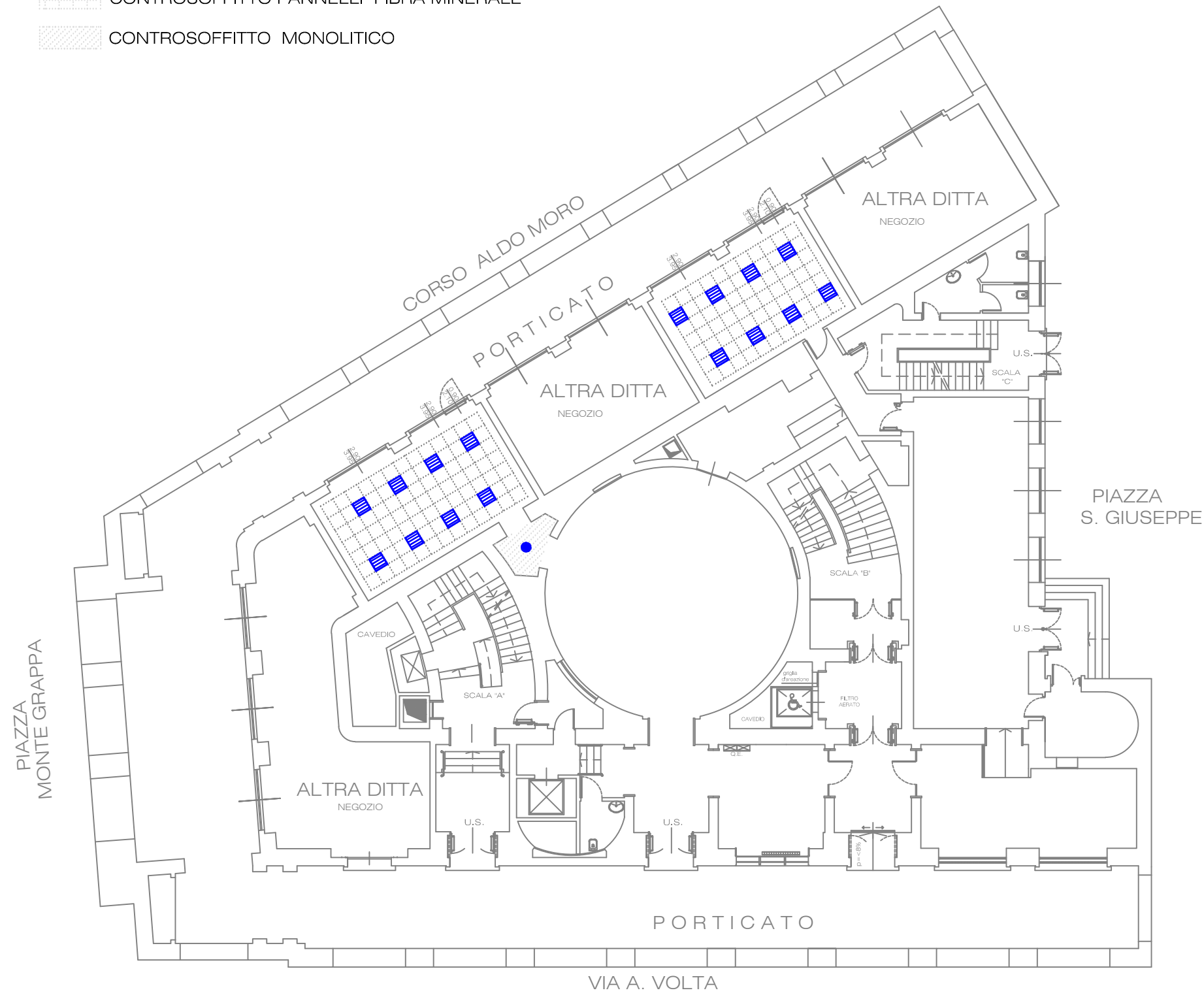
PIANTA PIANO TERRA (Quota 0.00) PIANTA CORPI ILLUMINANTI
