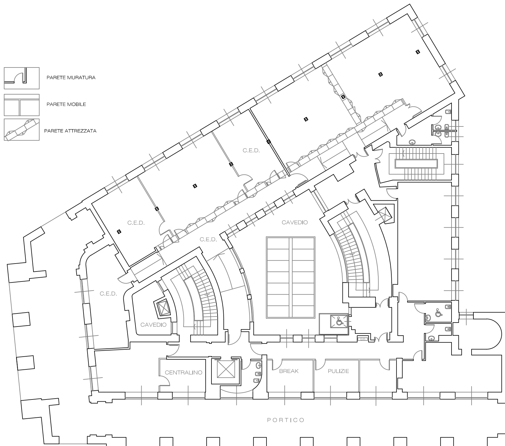
PIANTA PIANO AMMEZZATO (Quota +5.27 ) ALTEZZA PIANO = MT 3.45 SITUAZIONE ATTUALE
