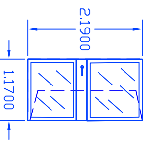
porta a vetro REI 60 con maniglione
