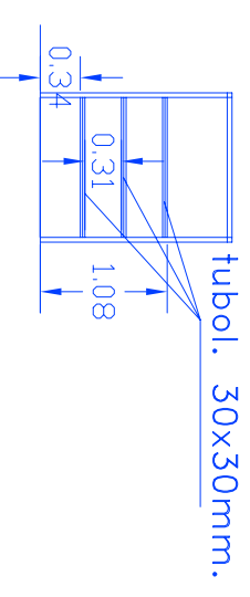
Controtelai finestre
