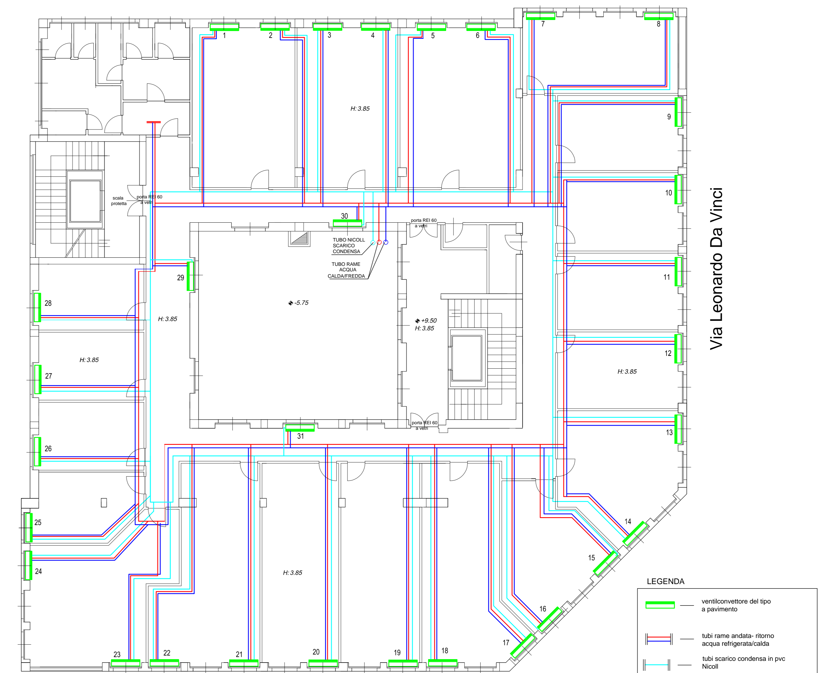
Pianta Piano Secondo Impianto di climatizzazione di progetto
