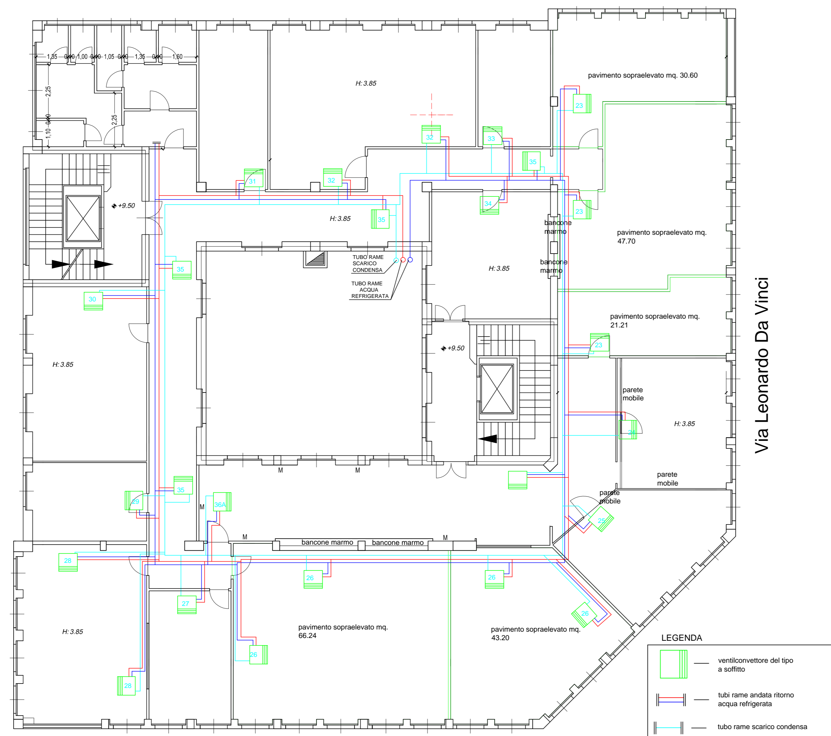
Pianta Piano Secondo Impianto di climatizzazione esistente
