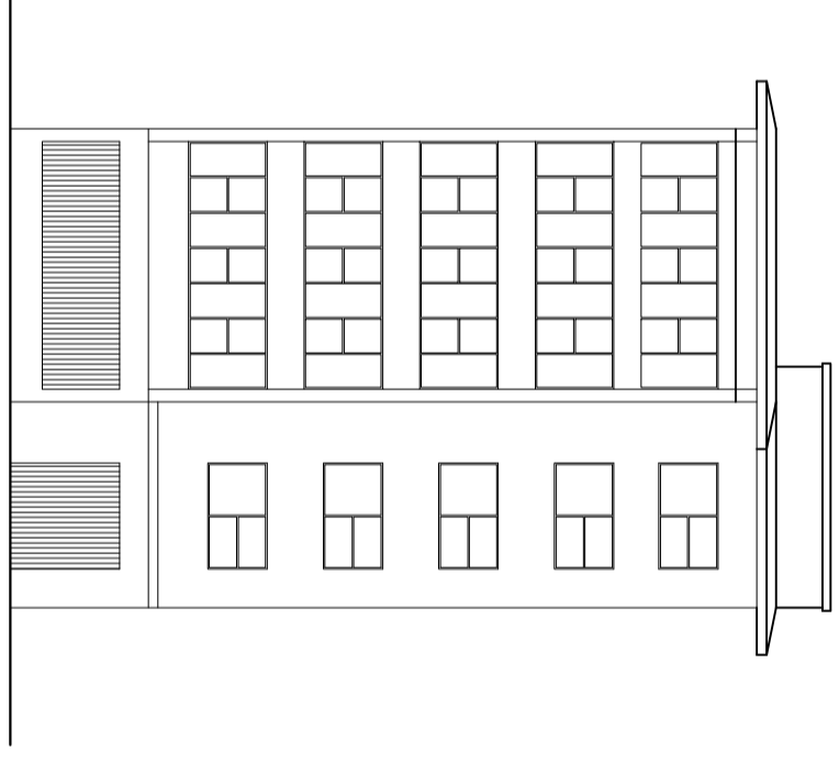
PROSPETTO EST - VIA MASIMO
