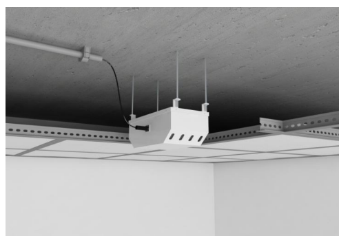
Fig. 1 Esempio di fissaggio a controsoffitto
