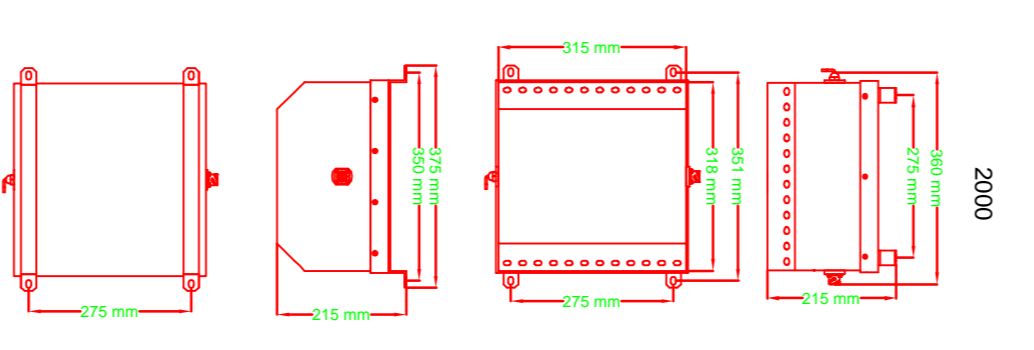
PARTICOLARI DIMENSIONALI DI MASSIMA GENERATORI AEROSOL
