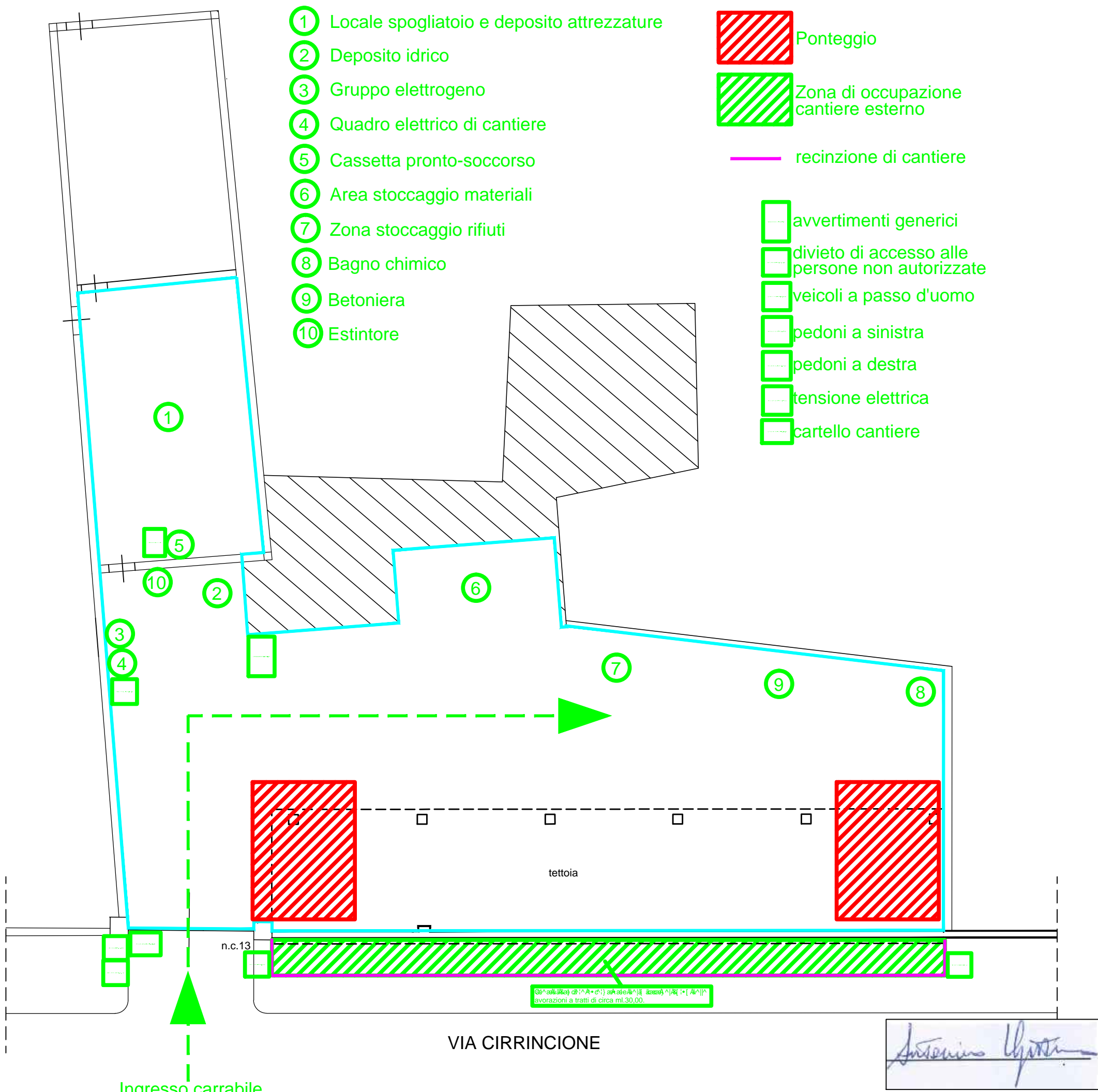
PLANIMETRIA DI CANTIERE scala 1:100
