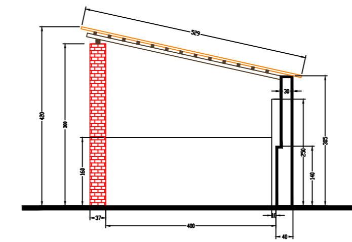
SEZIONE A-B Scala 1:50
