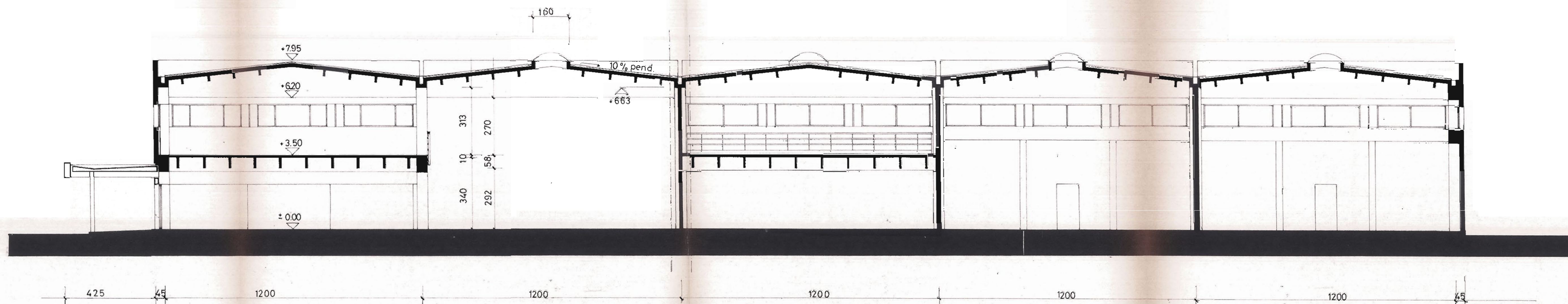
SEZIONE BB
