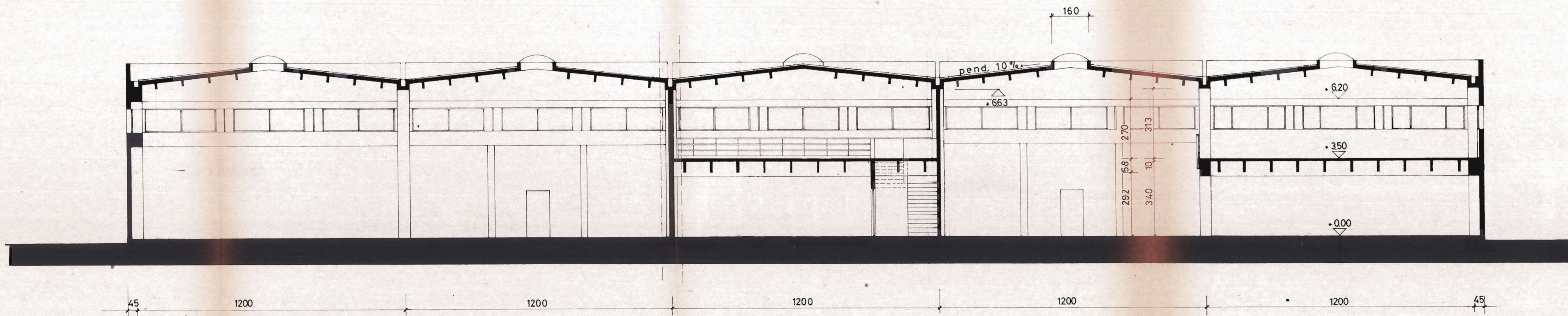
SEZIONE BB
