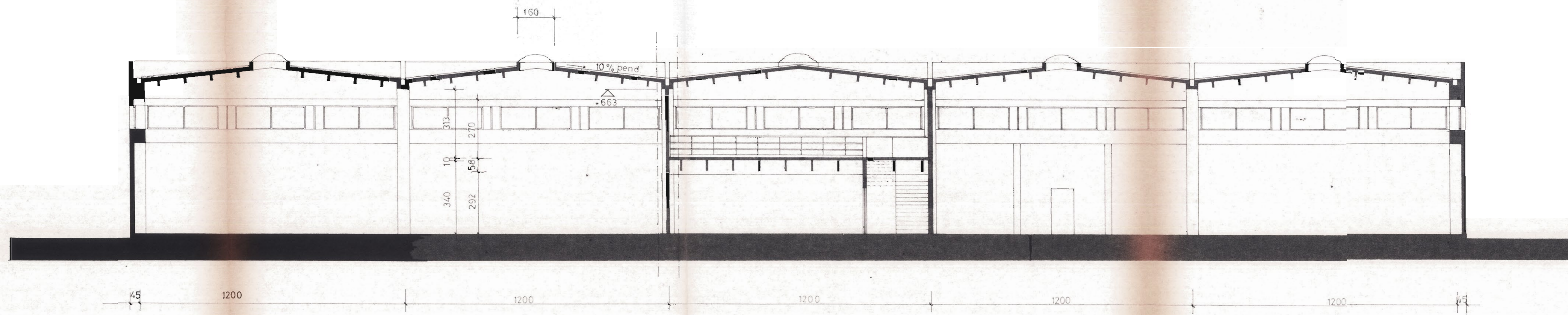
SEZIONE B-B
