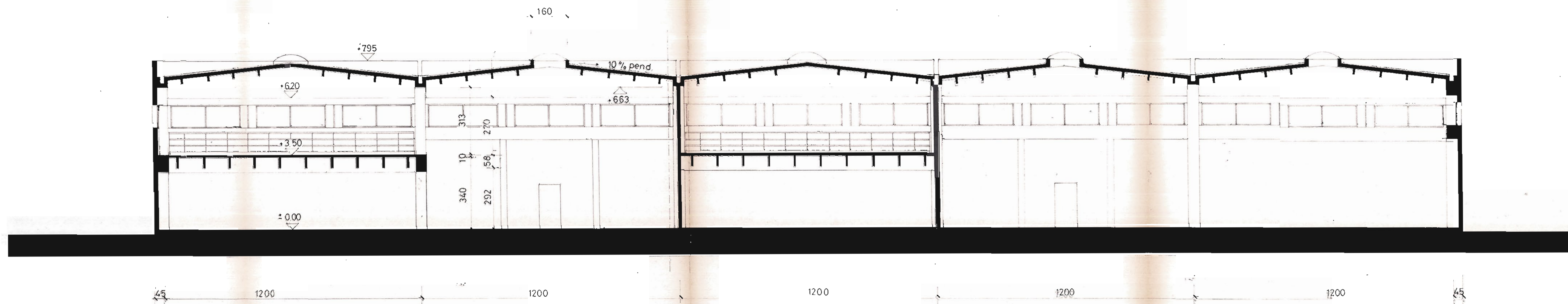
SEZIONE BB
