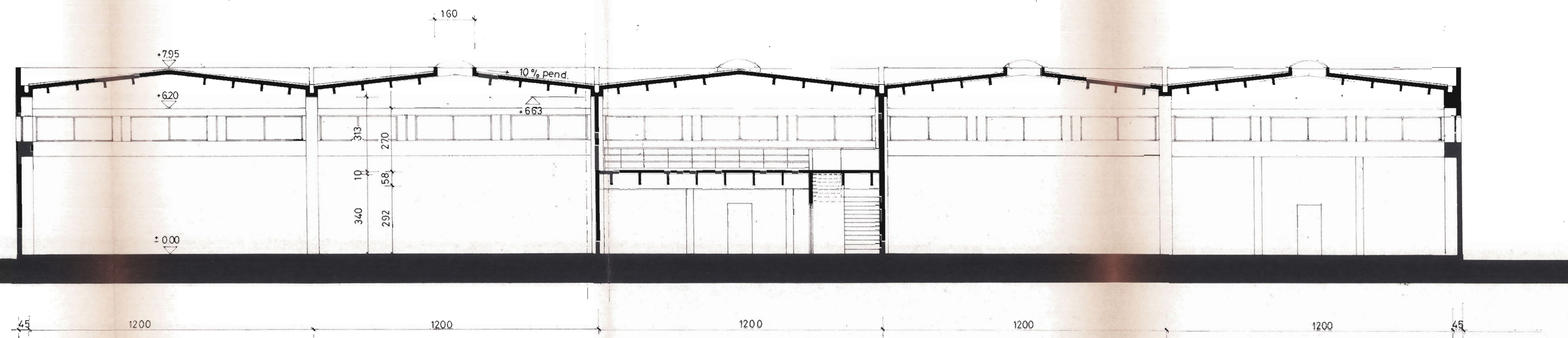
SEZIONE BB
