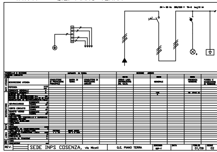
TAV. "A" - Q.E. PIANO TERRA
