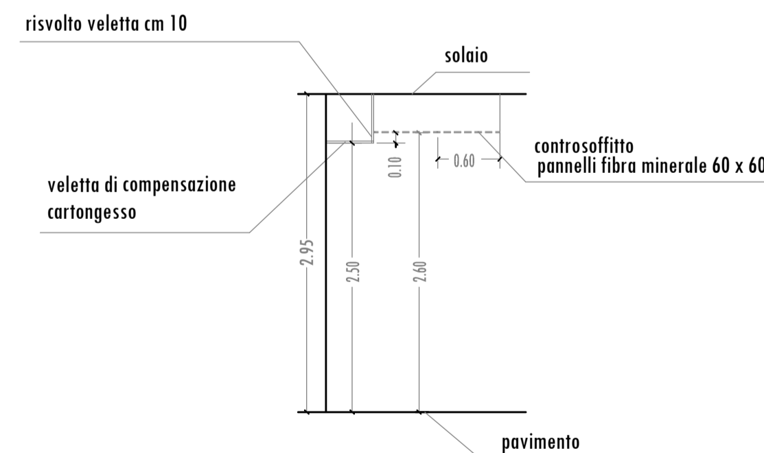
SEZIONE INDICATIVA A-A
