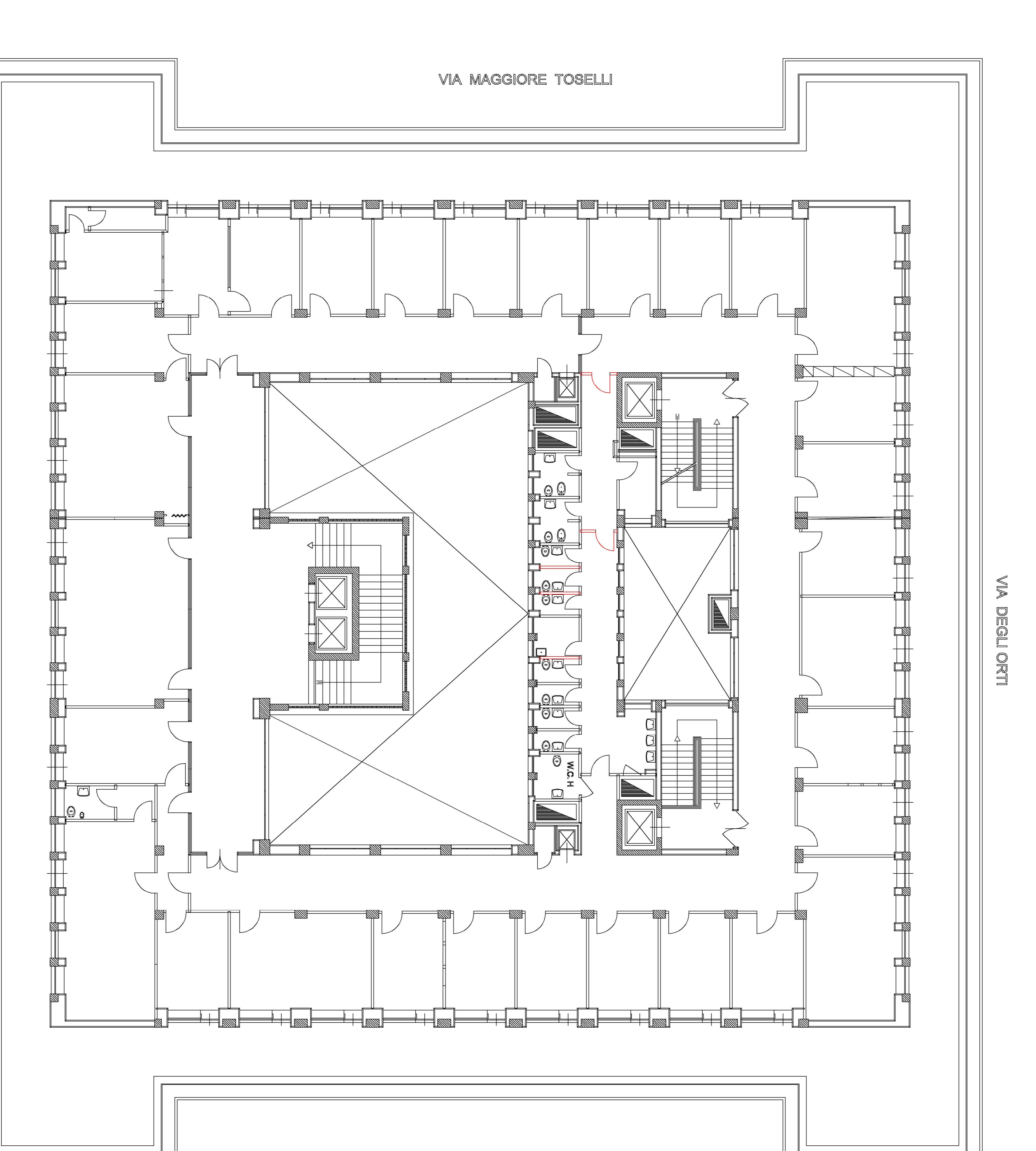
PIANO 6° STATO DI PROGETTO VIA LAURANA
