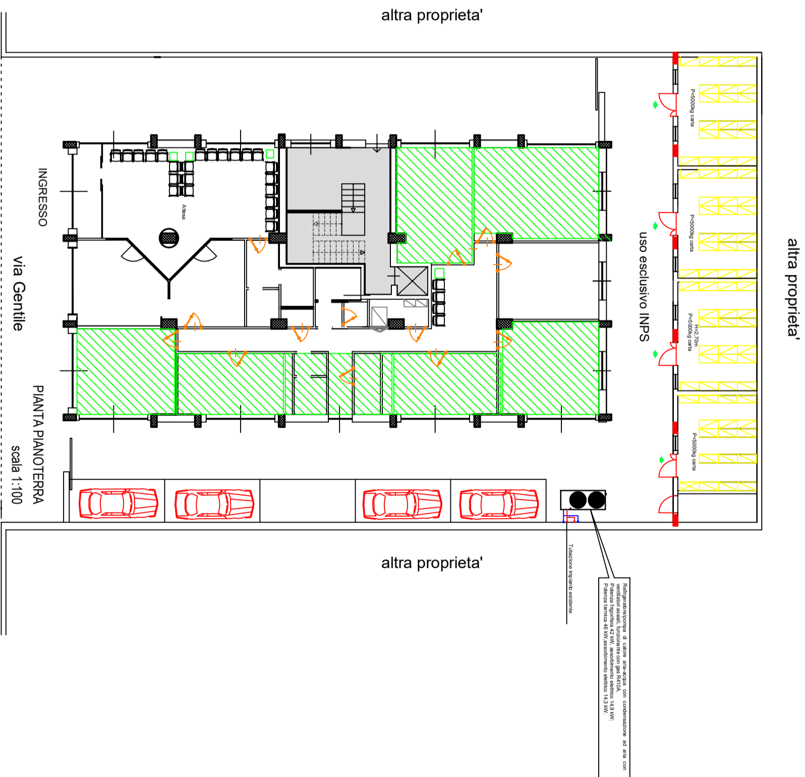
PIANIMETRIA scala 1:100
