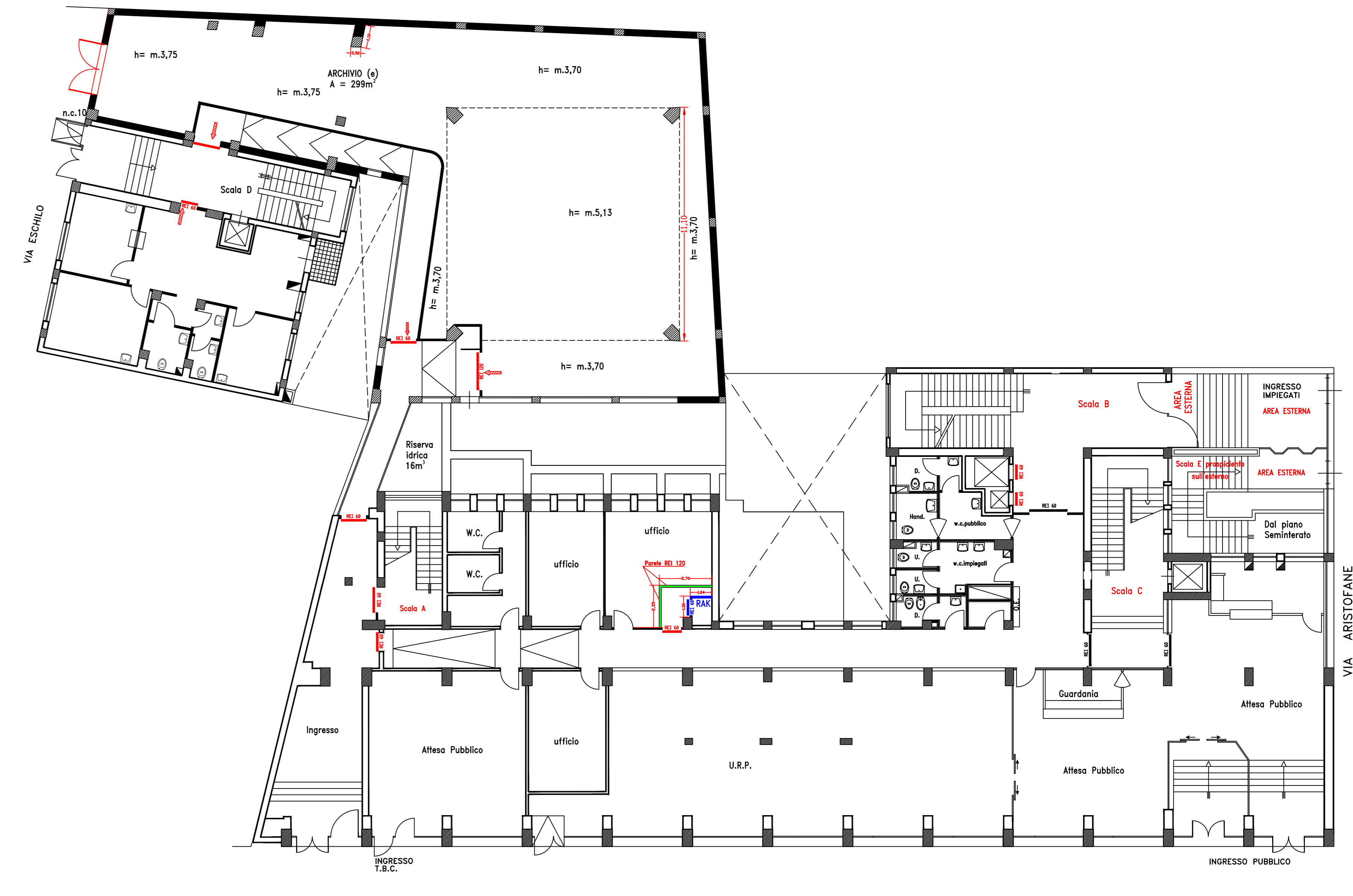
PIANO RIALZATO
