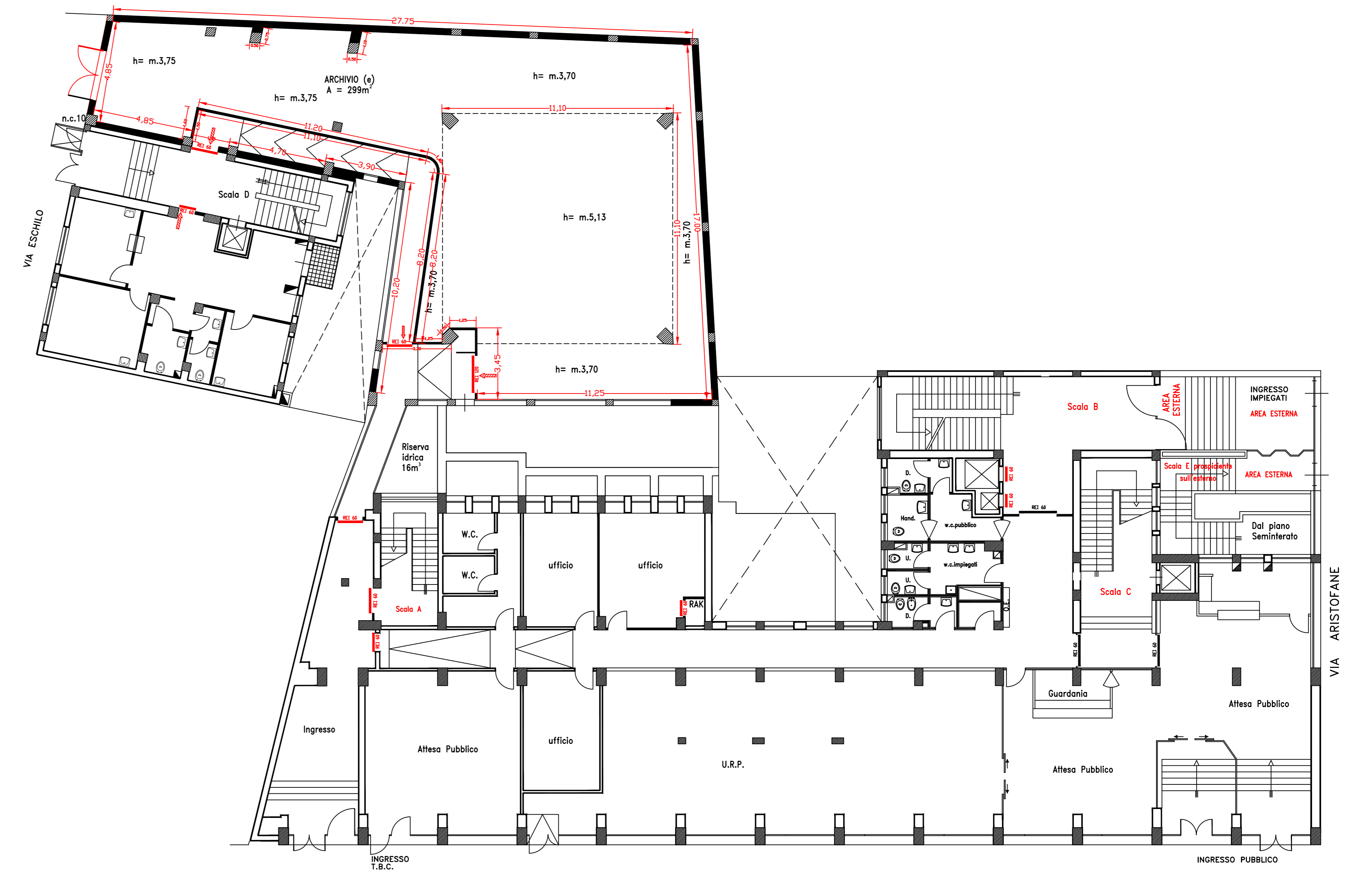
PIANO RIALZATO
