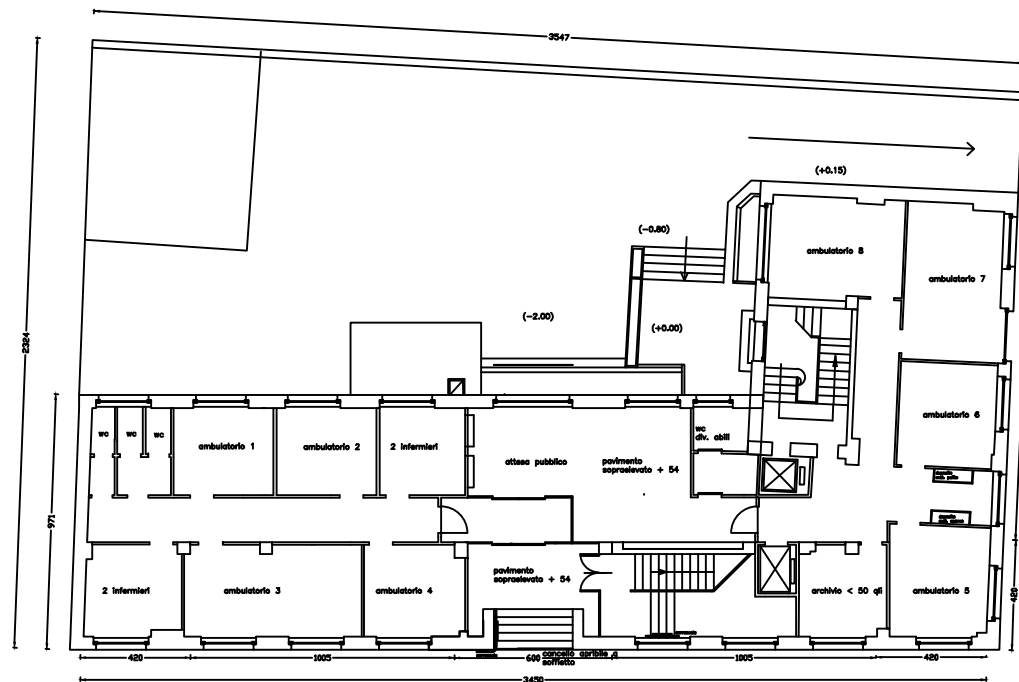
PIANTA PIANO RIALZATO STATO DI PROGETTO
